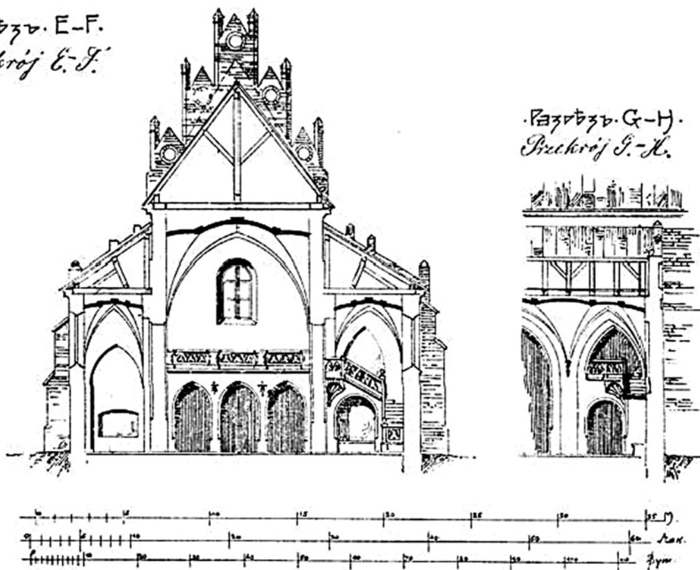
266. Ciechanów. Projekt restauracji fary Narodzenia NMP, przekrój, 1909
