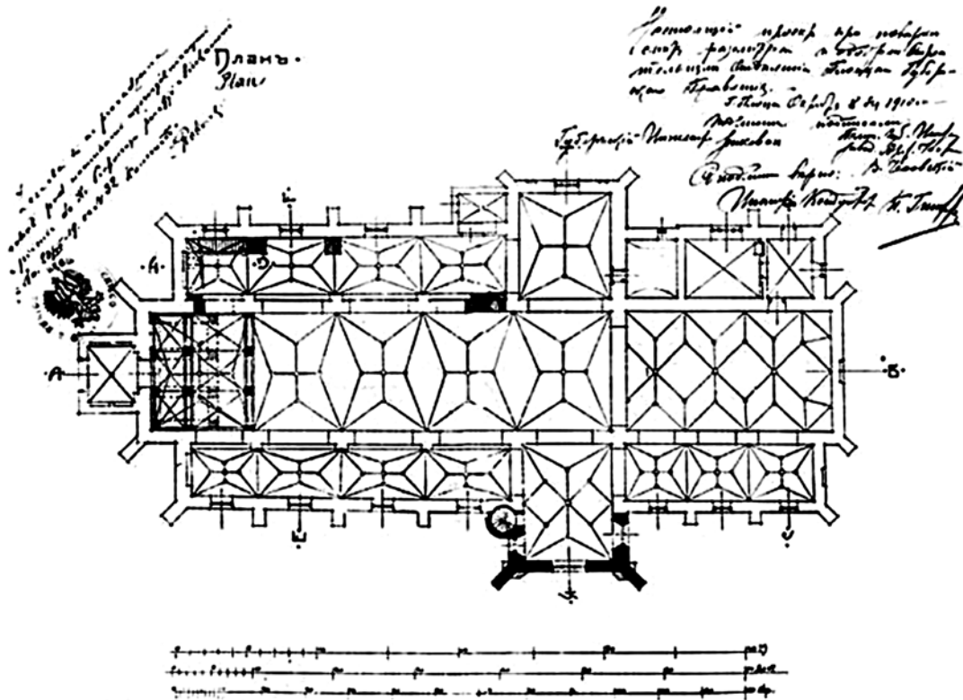
264. Ciechanów. Projekt restauracji fary Narodzenia NMP, rzut, 1909
